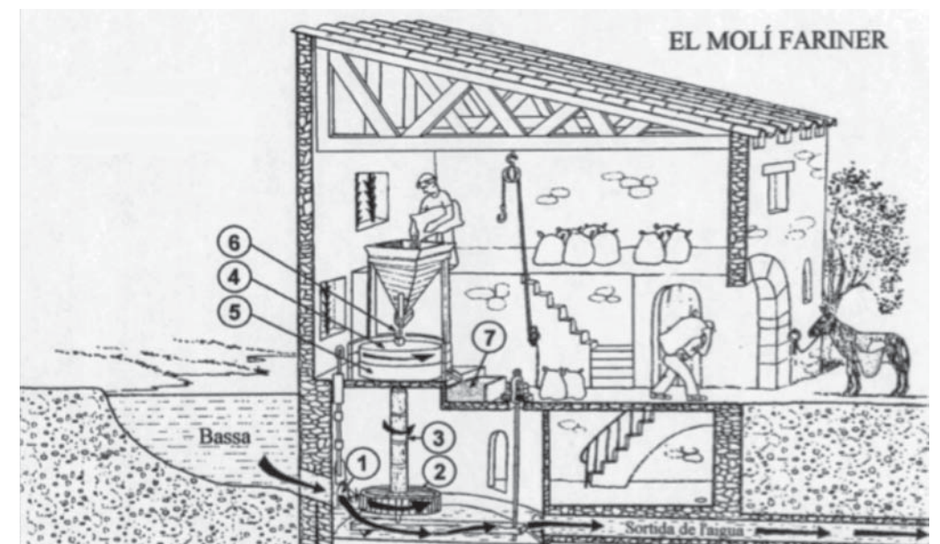
Esquema del funcionament d'un molí fariner
